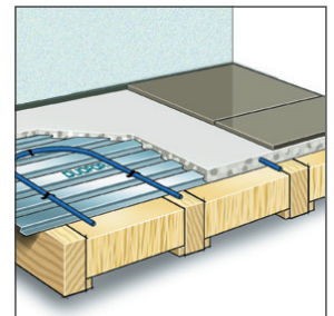
Vloer met vloerverwarming
