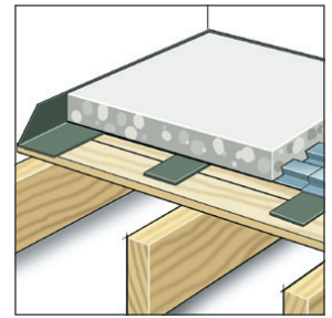
Geluidsisolerend op vloerdelen
