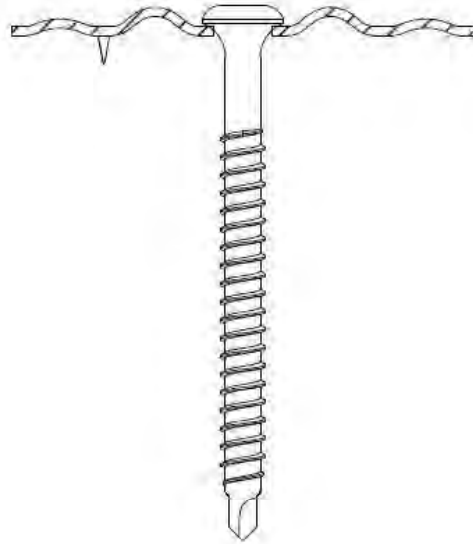
Eurofast EDS-SRB 4,8 x L
