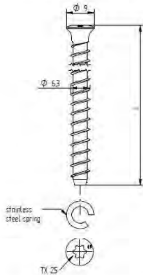
VRF Eurofast EAS 6,3 x L
