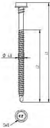
Eurofast EDS-BZTR/BGTR 4,8 x L
