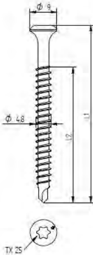
Eurofast EDS-B 4,8 x L
