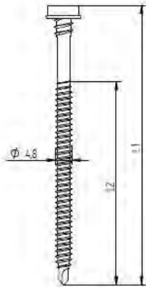
Eurofast EDS-BZT 4,8 x L
