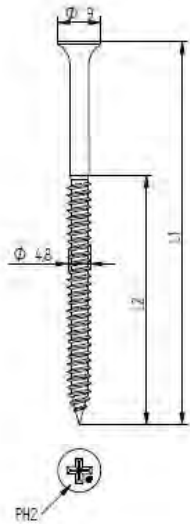
Eurofast EDS-S 4,8 x L
