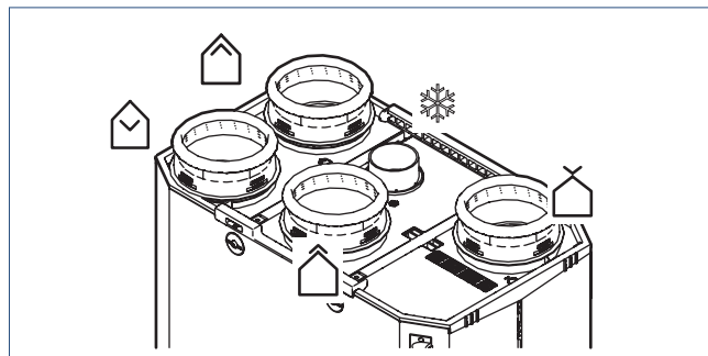
Aansluitingen bovenzijde
