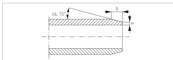
Abb. 4-3 Afschuiven van afgezaagde buisuiteinden
