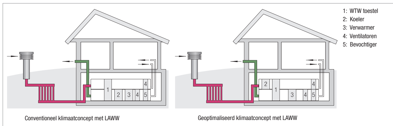
Afb. 3-5 Conventioneel en geoptimaliseerd klimaatconcept met LAWW
