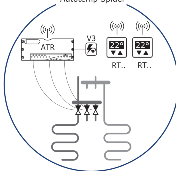
Detail: aansturing CV-circuits Autotemp Spider
